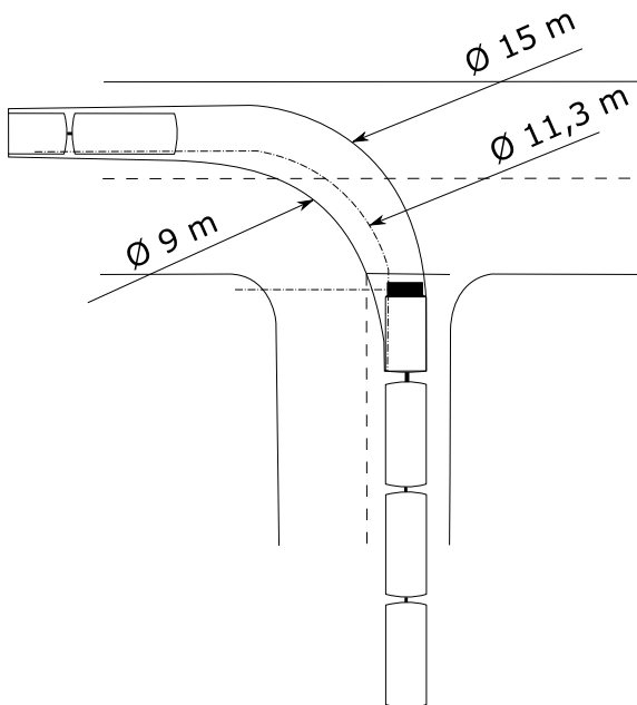
Schleppkurven-Darstellung
